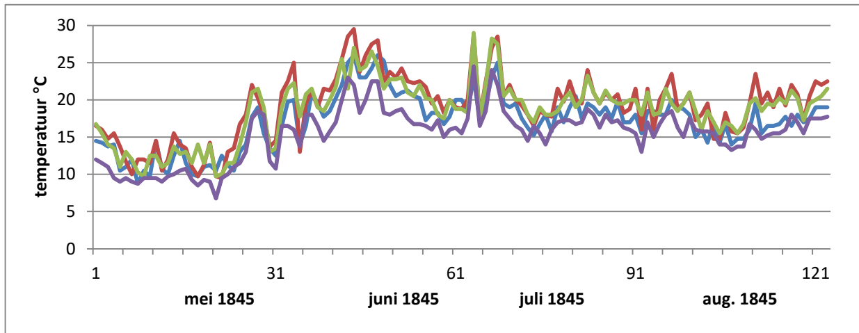
Fig. 1. Thermometrische waarnemingen verricht te Brugge door Louis Matthys voor de maanden mei, juni, juli en augustus 1845 op verschillende uren van de dag (Matthys, 1846).
